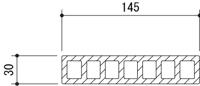
EP-A1503断面図
