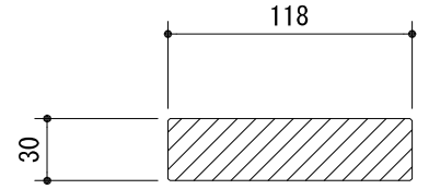
EP-M1203断面図
