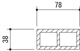
EP-A7838断面図
