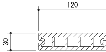
EP-A1203断面図
