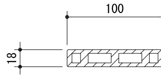
EP-A1018断面図
