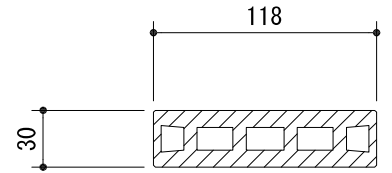
EP-LA1203断面図
