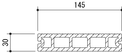
EP-LA1503断面図
